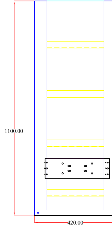
Yan Görünüş
