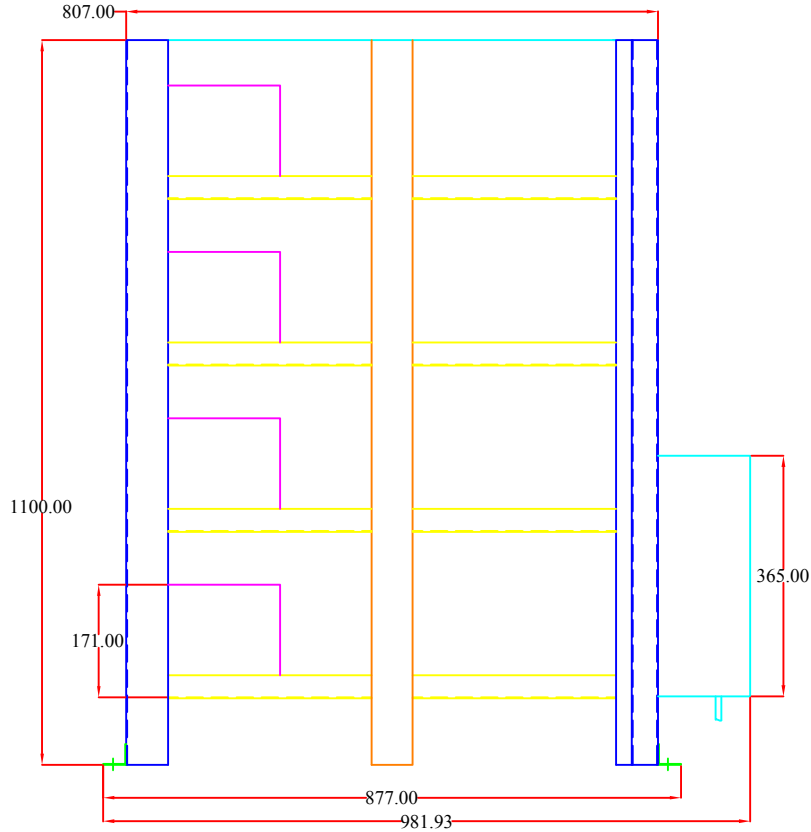
Ön Görünüş
