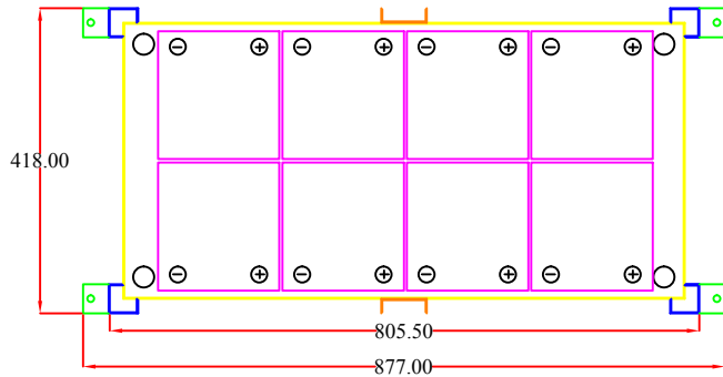
Üst Görünüş
