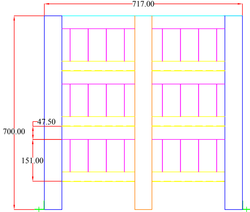
Ön Görünüş
